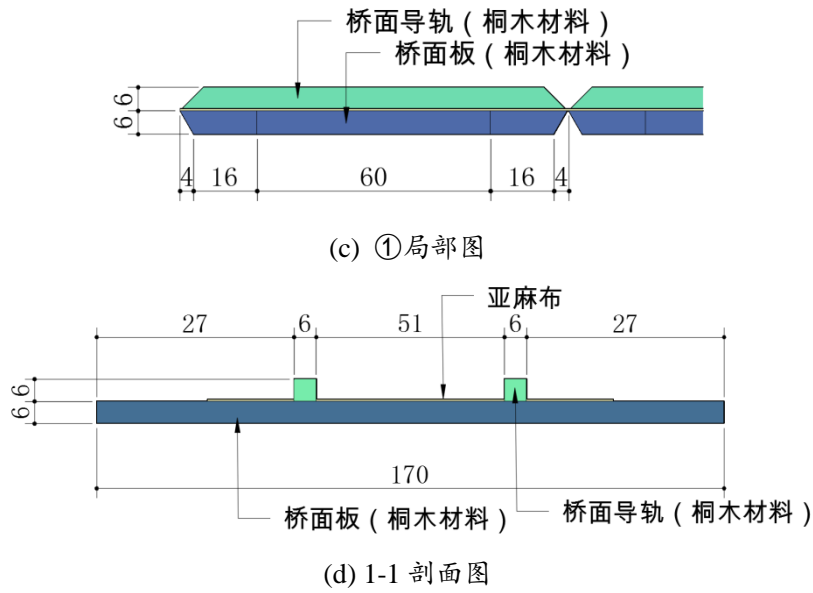
图6 桥面板详图
